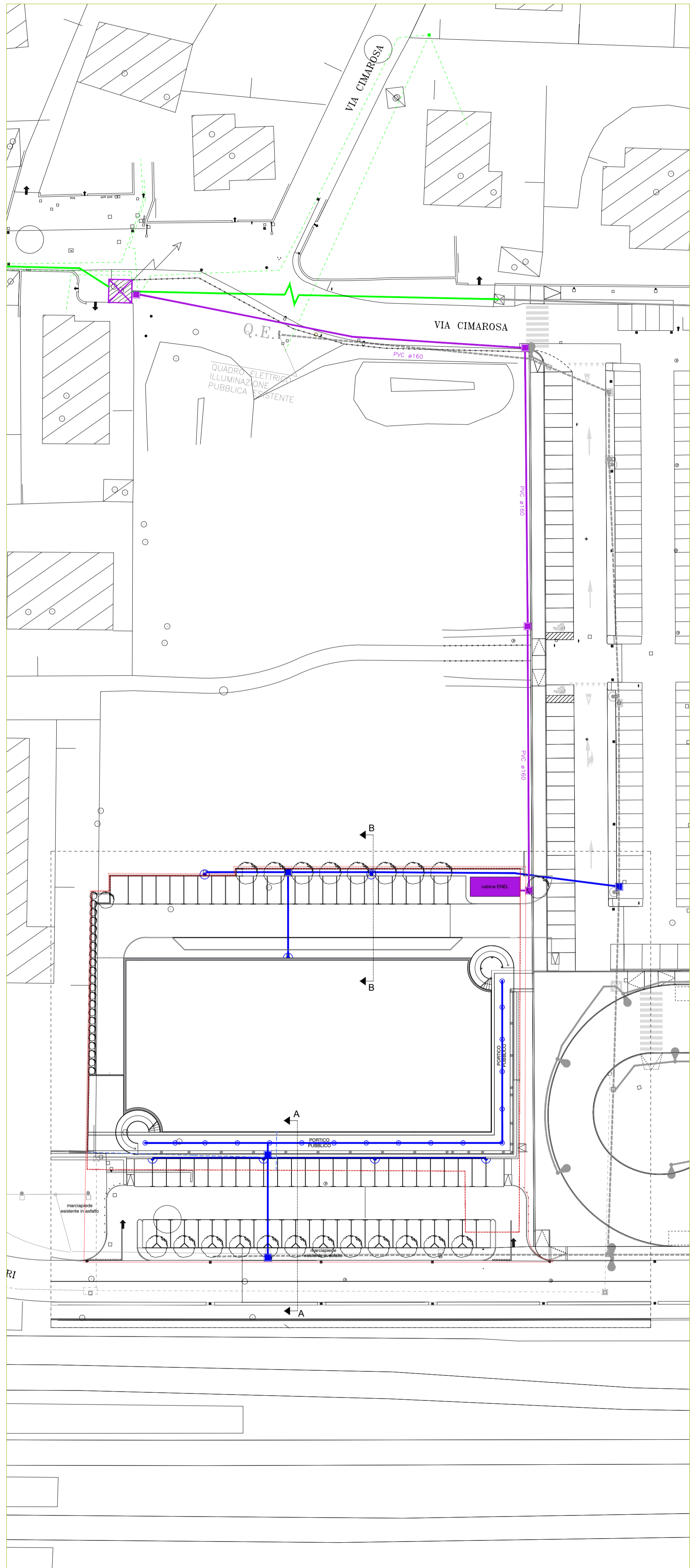
PLANIMETRIA DI INQUADRAMENTO Sc. 1:500
