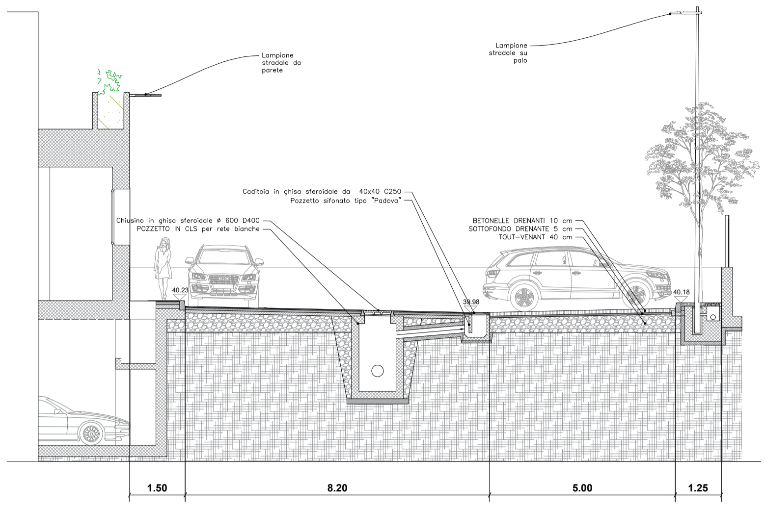
SEZIONE TIPO B-B Sc. 1:100
