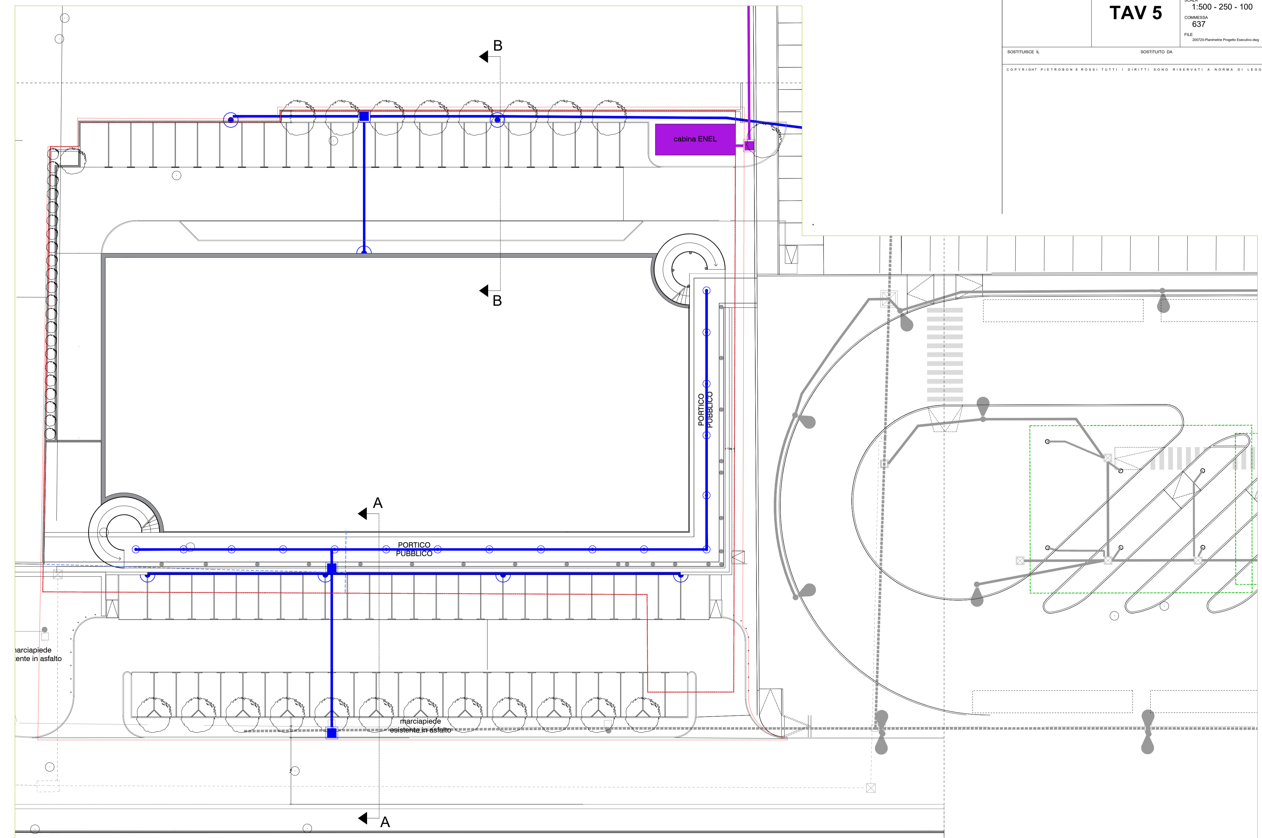
PLANIMETRIA DI DETTAGLIO Sc. 1:250
