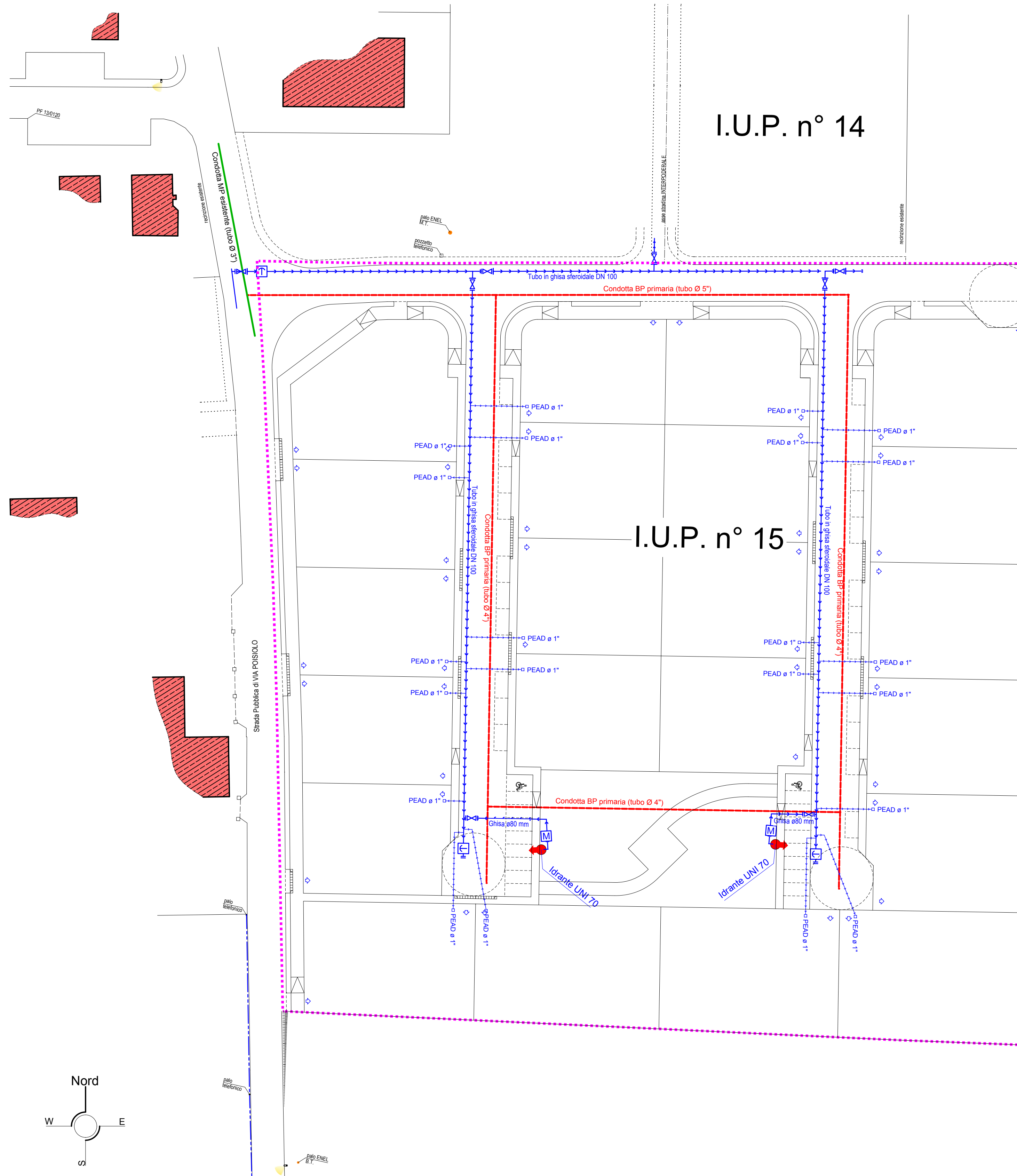
PLANIMETRIA SCALA 1: 500
